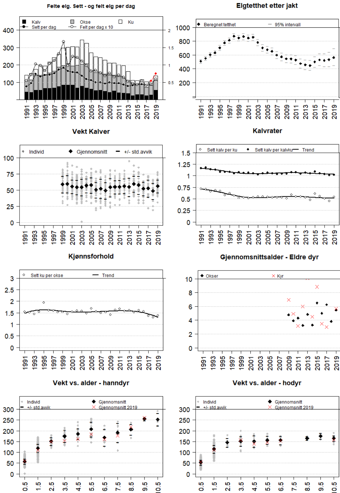
Figur Kviteseid. Felte elg, sett elg per jegerdag, samt felt elg per jegerdag*10 (øvre venstre delfigur), estimert elgtetthet (øvre høyre delfigur), gjennomsnittlige slaktevekt for kalv (nest overste venstre delfigur), kalve- og tvillingrate (nest overste høyre delfigur), sett ku per okse (nest nederste venstre delfigur), gjennomsnittsalder for eldre dyr 2,5 år eller eldre (nest nederste høyre delfigur), vektutvikling i forhold til årsklasse for hanndyr (nedre venstre delfigur) og hodyr (nedre høyre delfigur).
