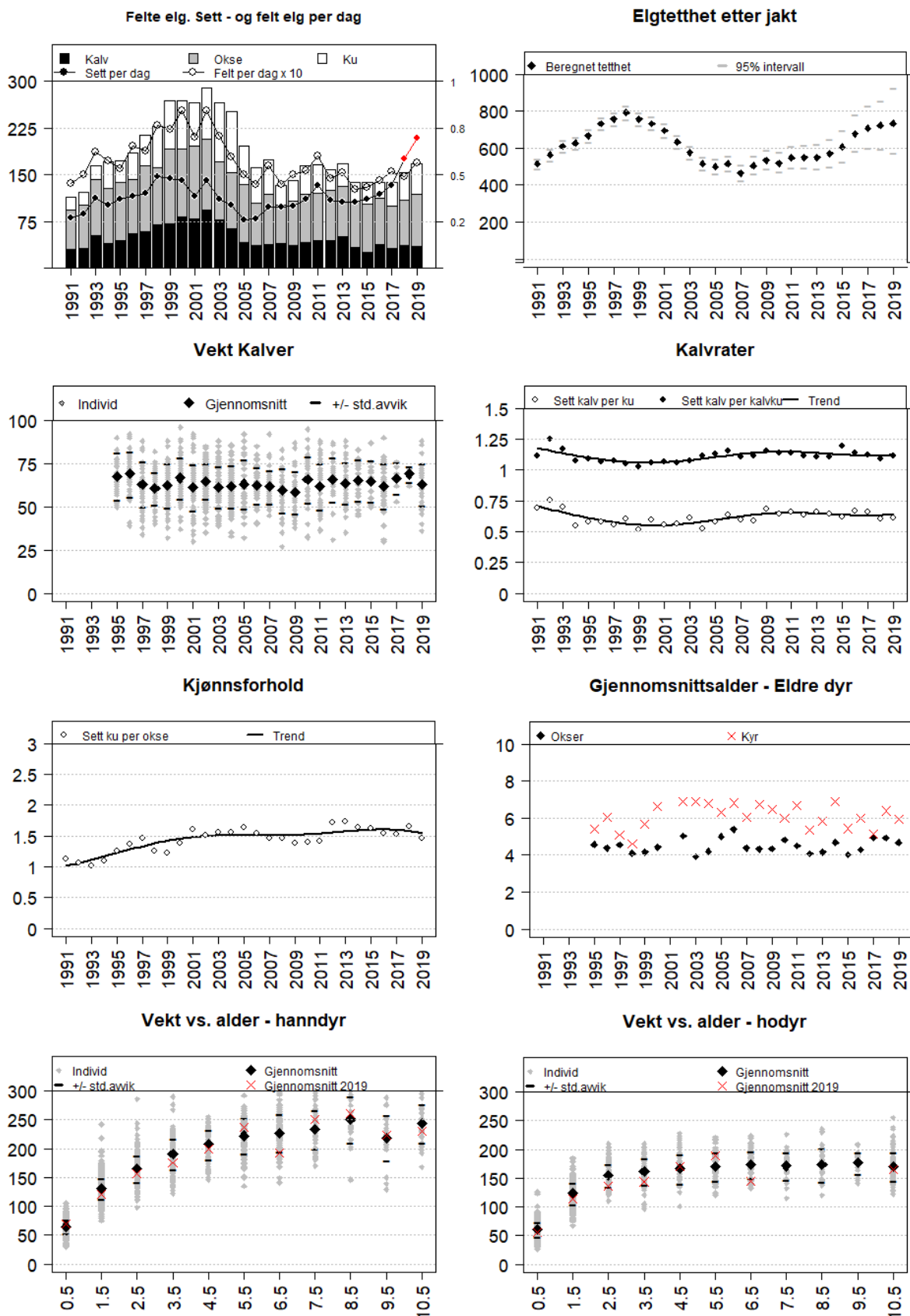
Figur Vinje. Felte elg, sett elg per jegerdag, samt felt elg per jegerdag*10 (øvre venstre delfigur), estimert elgtetthet (øvre høyre delfigur), gjennomsnittlige slaktevekt for kalv (nest øverste venstre delfigur), kalve- og tvillingrate (nest øverste høyre delfigur), sett ku per okse (nest nederste venstre delfigur), gjennomsnittsalder for eldre dyr 2,5 år eller eldre (nest nederste høyre delfigur), vektutvikling i forhold til årsklasse for hanndyr (nedre venstre delfigur) og hodyr (nedre høyre delfigur).
