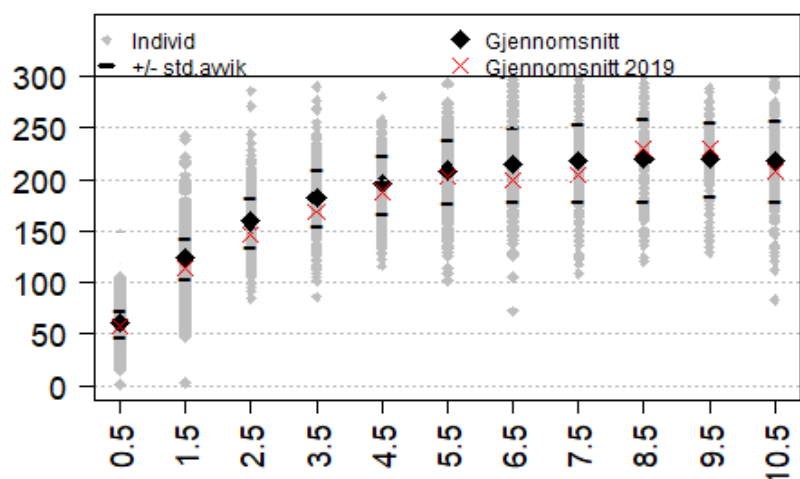
Figur 11. Gjennomsnittsvækt i forhold til alder for okser skutt i Telemark i perioden 1992-2019 med svarte ruter (n=20 982). Svarte streker viser øvre og nedre grense for 95 % konfidensintervall for forventet vekt til de samme aldersklassene. Enkeltindivider vist med grå punkter og gjennomsnittlig vekt for okser felt i 2019 (n=810) vist med røde kryss.
