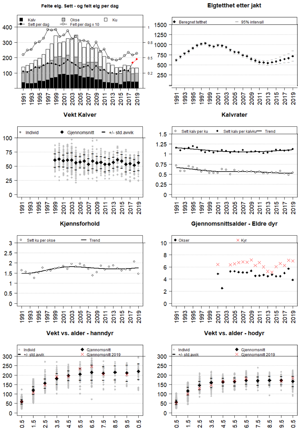
Figur Fyresdal. Felte elg, sett elg per jegerdag, samt felt elg per jegerdag*10 (øvre venstre delfigur), estimert elgtetthet (øvre høyre delfigur), gjennomsnittlige slaktevekt for kalv (nest øverste venstre delfigur), kalve- og tvillingrate (nest øverste høyre delfigur), sett ku per okse (nest nederste venstre delfigur), gjennomsnittsalder for eldre dyr 2,5 år eller eldre (nest nederste høyre delfigur), vektutvikling i forhold til årsklasse for hanndyr (nedre venstre delfigur) og hodyr (nedre høyre delfigur).
