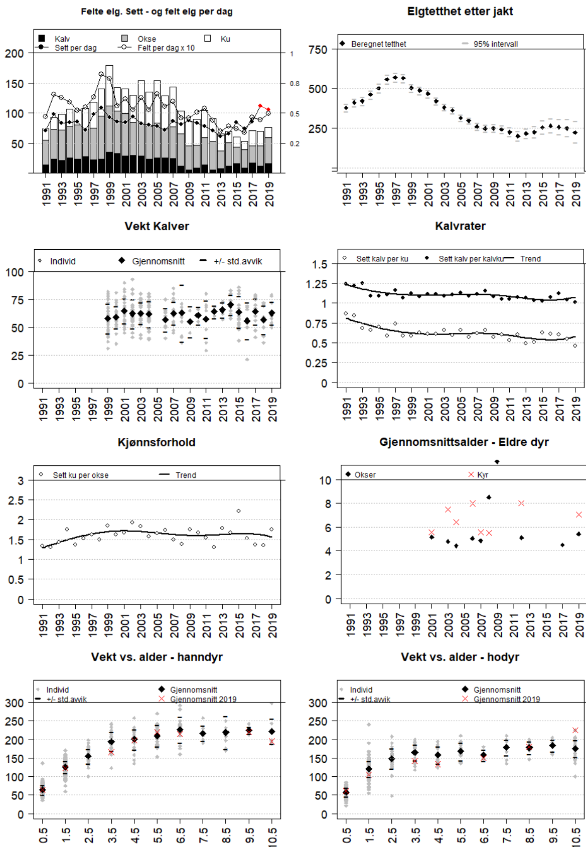
Figur Seljord. Felte elg, sett elg per jegerdag, samt felt elg per jegerdag*10 (øvre venstre delfigur), estimert elgtetthet (øvre høyre delfigur), gjennomsnittlige slaktevekt for kalv (nest øverste venstre delfigur), kalve- og tvillingrate (nest øverste høyre delfigur), sett ku per okse (nest nederste venstre delfigur), gjennomsnittsalder for eldre dyr 2,5 år eller eldre (nest nederste høyre delfigur), vektutvikling i forhold til årsklasse for hanndyr (nedre venstre delfigur) og bodyr (nedre høyre delfigur).
