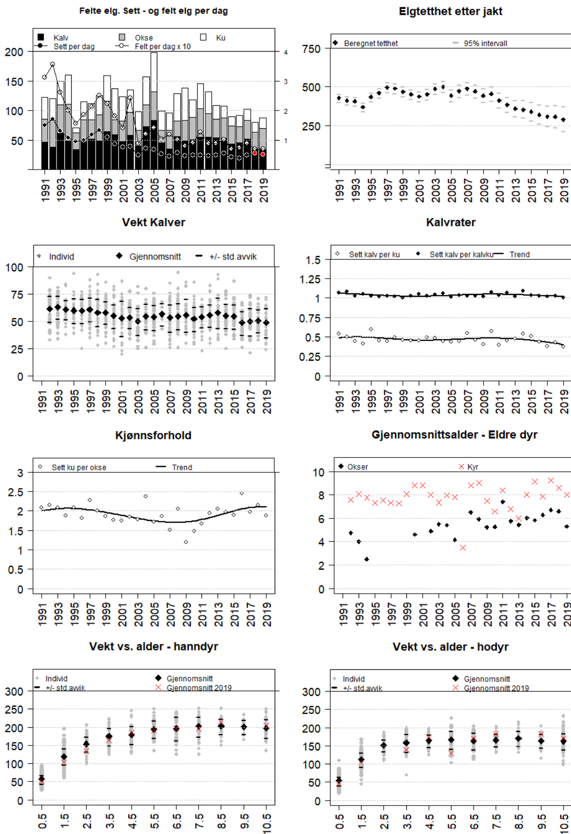
Figur Siljan. Felte elg, sett elg per jegerdag, samt felt elg per jegerdag*10 (øvre venstre delfigur), estimert elgtetthet (øvre høyre delfigur), gjennomsnittlige slaktevekter for kalv (nest øverste venstre delfigur), kalve- og tvillingrate (nest øverste høyre delfigur), sett ku per okse (nest nederste venstre delfigur), gjennomsnittsalder for eldre dyr 2,5 år eller eldre (nest nederste høyre delfigur), vektutvikling i forhold til årsklasse for hanndyr (nedre venstre delfigur) og hodyr (nedre høyre delfigur).
