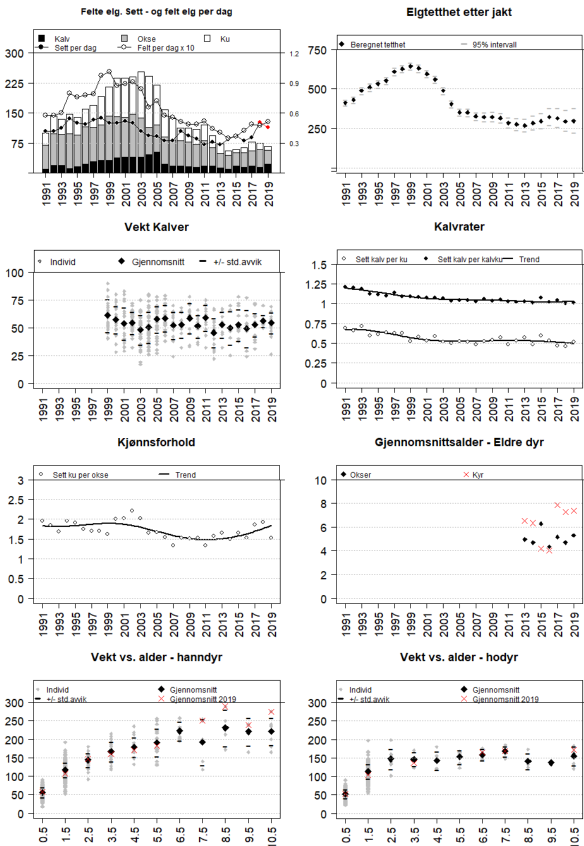
Figur Nissedal. Felte elg, sett elg per jegerdag, samt felt elg per jegerdag*10 (øvre venstre delfigur), estimert elgtetthet (øvre høyre delfigur), gjennomsnittlige slaktevekt for kalv (nest overste venstre delfigur), kalve- og trillingrate (nest overste høyre delfigur), sett ku per okse (nest nederste venstre delfigur), gjennomsnittsalder for eldre dyr 2,5 år eller eldre (nest nederste høyre delfigur), vektutvikling i forhold til årsklasse for hanndyr (nedre venstre delfigur) og hodyr (nedre høyre delfigur).
