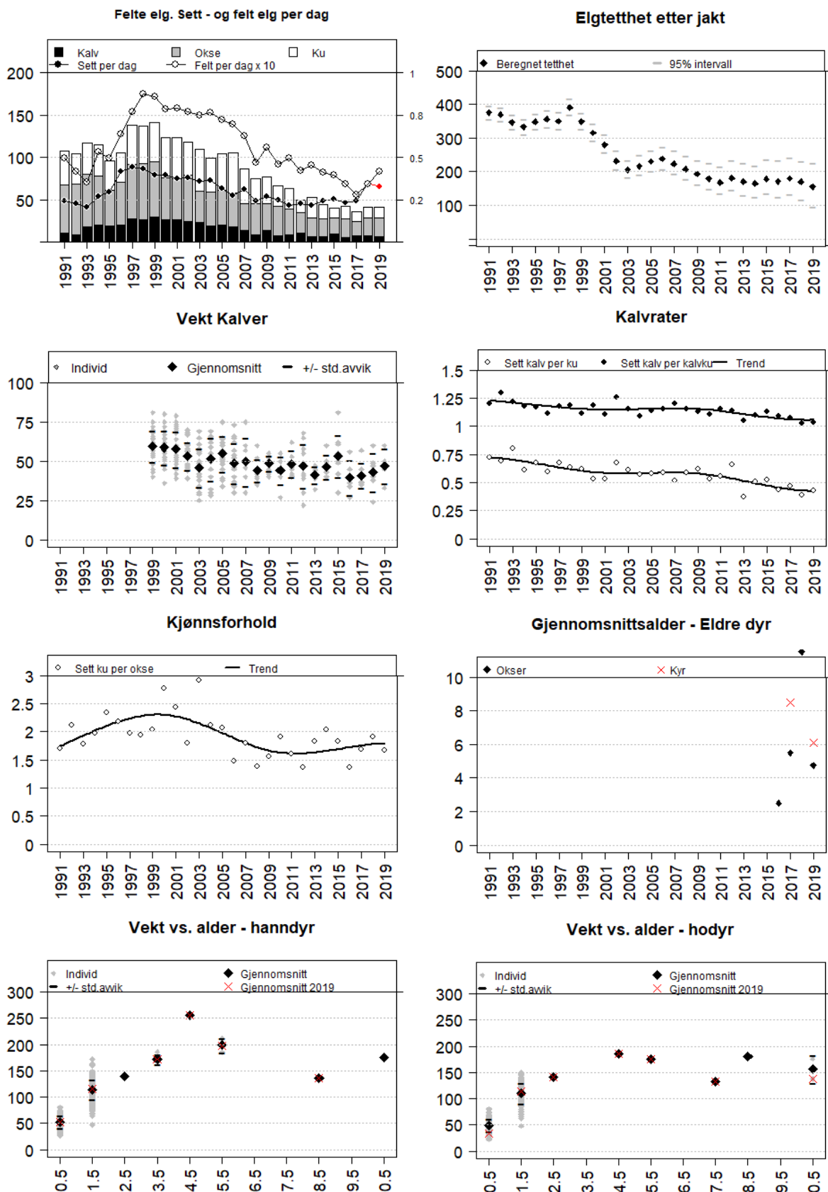
Figur Kragerø. Felte elg, sett elg per jegerdag, samt felt elg per jegerdag*10 (øvre venstre delfigur), estimert elgtetthet (øvre høyre delfigur), gjennomsnittlige slaktevekt for kalv (nest øverste venstre delfigur), kalve- og tvillingrate (nest øverste høyre delfigur), sett ku per okse (nest nederste venstre delfigur), gjennomsnittsalder for eldre dyr 2,5 år eller eldre (nest nederste høyre delfigur), vektutvikling i forhold til årsklasse for hanndyr (nedre venstre delfigur) og hodyr (nedre høyre delfigur).
