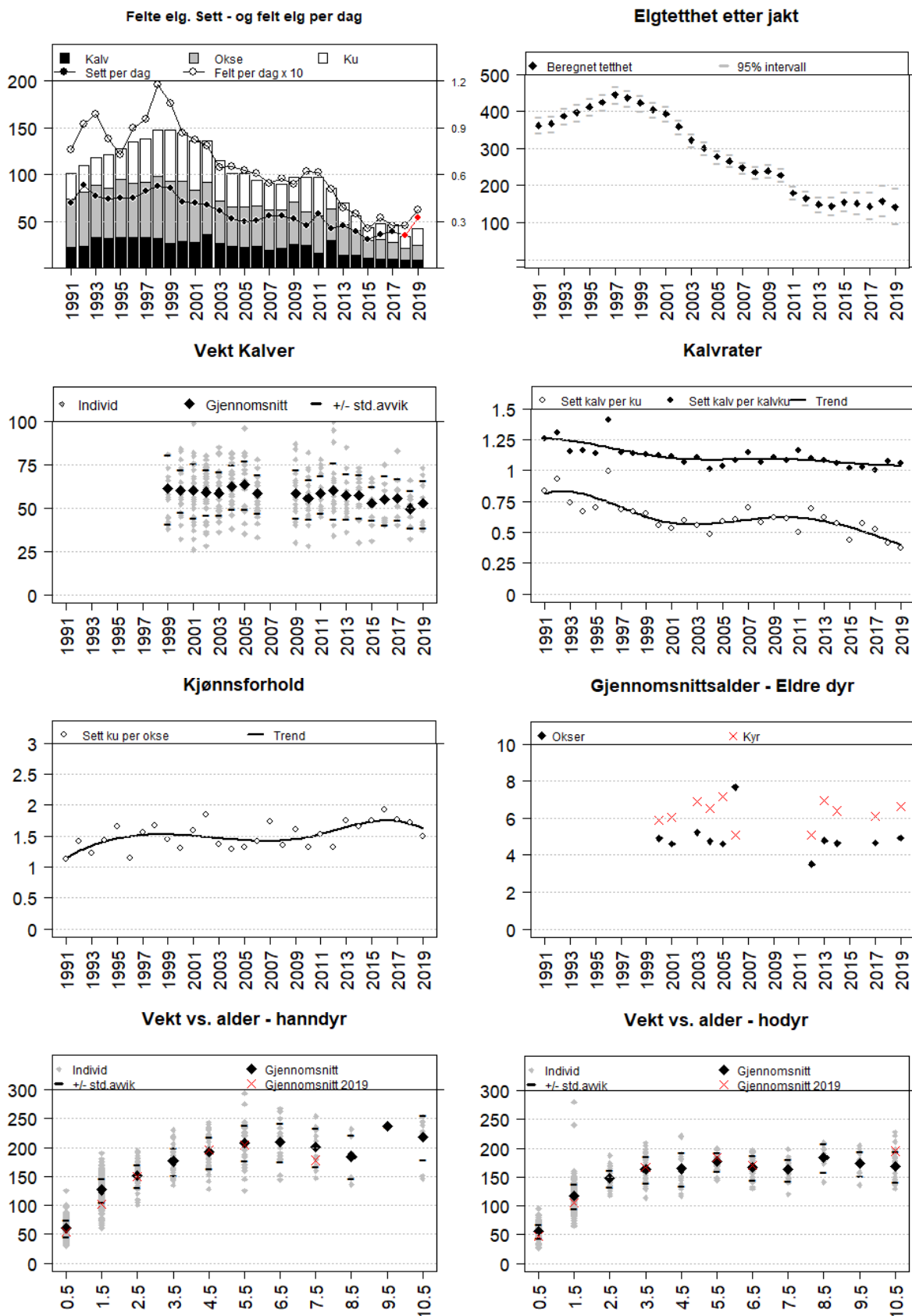
Figur Sauherad. Felte elg, sett elg per jegerdag, samt felt elg per jegerdag*10 (øvre venstre delfigur), estimert elgtetthet (øvre høyre delfigur), gjennomsnittlige slaktevekt for kalv (nest øvre venstre delfigur), kalve- og tvillingrate (nest øvre høyre delfigur), sett ku per okse (nest nederste venstre delfigur), gjennomsnittsalder for eldre dyr 2,5 år eller eldre (nest nederste høyre delfigur), vektutvikling i forhold til årsklasse for hanndyr (nedre venstre delfigur) og hodyr (nedre høyre delfigur).
