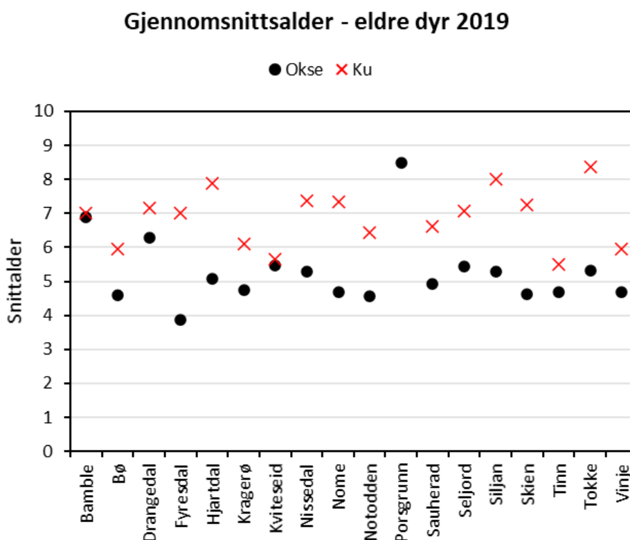
Figur 14. Gjennomsnittlig alder for felte kyr (røde kryss) og okser (svarte punkter) minst 2,5 år gamle felt i kommuner i Telemark i 2019. Merk at det er betydelig variasjon i antall observasjoner per kommune. For eksempel består «snittalderen» i Porsgrunn kun av 1 okse (8,5 år) og 1 kyr (13,5 år).
