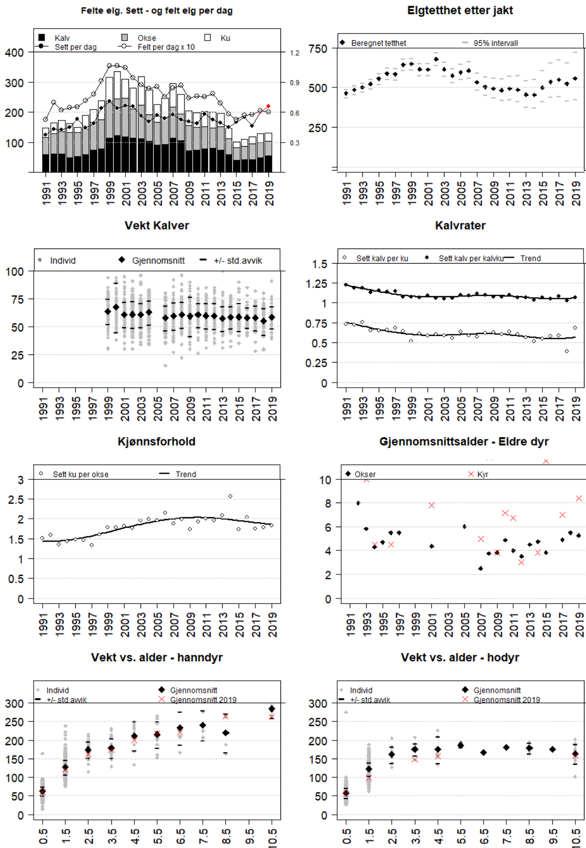
Figur Tokke. Felte elg, sett elg per jegerdag, samt felt elg per jegerdag*10 (øvre venstre delfigur), estimert elgtetthet (øvre høyre delfigur), gjennomsnittlige slaktevekt for kalv (nest overste venstre delfigur), kalve- og trillingrate (nest overste høyre delfigur), sett ku per okse (nest nederste venstre delfigur), gjennomsnittsalder for eldre dyr 2,5 år eller eldre (nest nederste høyre delfigur), vektutvikling i forhold til årsklasse for hanndyr (nedre venstre delfigur) og bodyr (nedre høyre delfigur).
