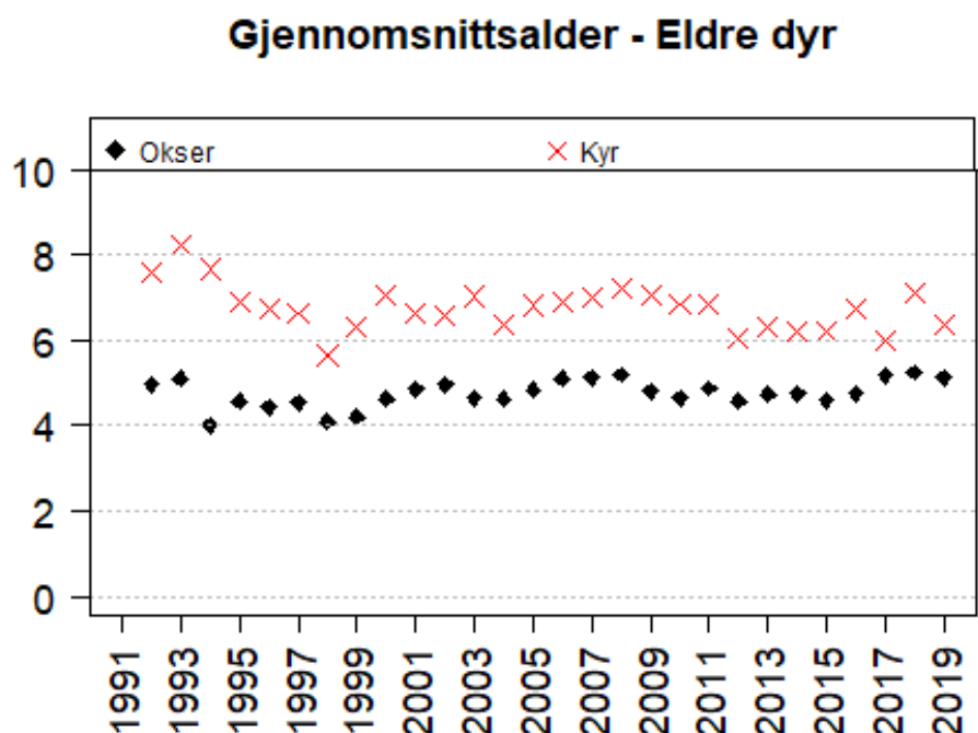
Figur 13. Gjennomsnittsalder for felte kyr (røde kryss, n=4731 ) og okser (svarte punkter, n=5190 ) minst 2,5 år gamle felt i Telemark i perioden 1992-2019.
