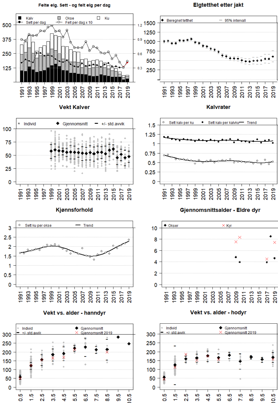
Figur Skien. Felte elg, sett elg per jegerdag, samt felt elg per jegerdag*10 (øvre venstre delfigur), estimert elgtetthet (øvre høyre delfigur), gjennomsnittlige slaktevekt for kalv (nest overste venstre delfigur), kalve- og trillingrate (nest overste høyre delfigur), sett ku per okse (nest nederste venstre delfigur), gjennomsnittsalder for eldre dyr 2,5 år eller eldre (nest nederste høyre delfigur), vektutvikling i forhold til årsklasse for hanndyr (nedre venstre delfigur) og hodyr (nedre høyre delfigur).
