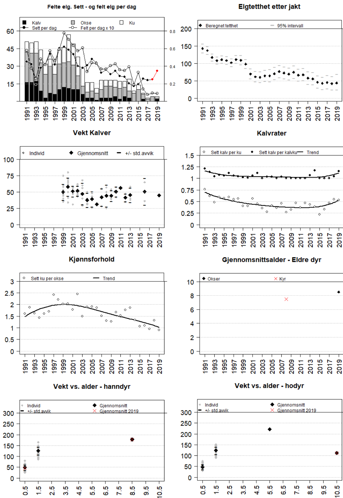
Figur Porsgrunn. Felte elg, sett elg per jegerdag, samt felt elg per jegerdag*10 (øvre venstre delfigur), estimert elgtetthet (øvre høyre delfigur), gjennomsnittlige slaktevekte for kalv (nest øvre venstre delfigur), kalve- og tvillingrate (nest øvre høyre delfigur), sett ku per okse (nest nederste venstre delfigur), gjennomsnittsalder for eldre dyr 2,5 år eller eldre (nest nederste høyre delfigur), vektutvikling i forhold til årsklasse for hanndyr (nedre venstre delfigur) og hodyr (nedre høyre delfigur).
