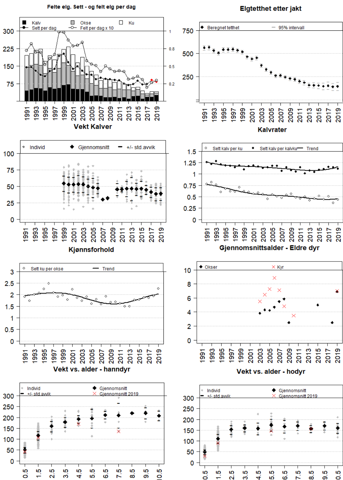
Figur Bamble. Felte elg, sett elg per jegerdag, samt felt elg per jegerdag*10 (øvre venstre delfigur), estimert elgtetthet (øvre høyre delfigur), gjennomsnittlige slaktevekt for kalv (nest øvre venstre delfigur), kalve- og tvillingrate (nest øvre høyre delfigur), sett ku per okse (nest nederste venstre delfigur), gjennomsnittsalder for eldre dyr 2,5 år eller eldre (nest nederste høyre delfigur), vektutvikling i forhold til årsklasse for hanndyr (nedre venstre delfigur) og bodyr (nedre høyre delfigur).
