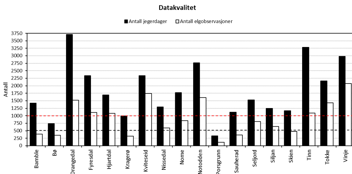
Figur 2. Antall jegerdager (svarte søyler), samt antall elgobservasjoner (hvite søyler) per kommune i Telemark i 2019. Rød stiple linje og svart stiple linje indikerer anbefalt «grense» over hhv. antall jegerdager og antall observasjoner av elg for at resultatene skal være statistisk sikre.
