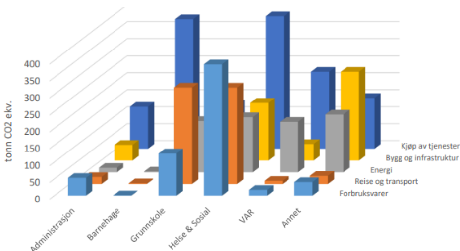
Figur 40 Klimafotavtrykk for Sauherad kommune si verksemd i 2016 (Asplan Viak)
