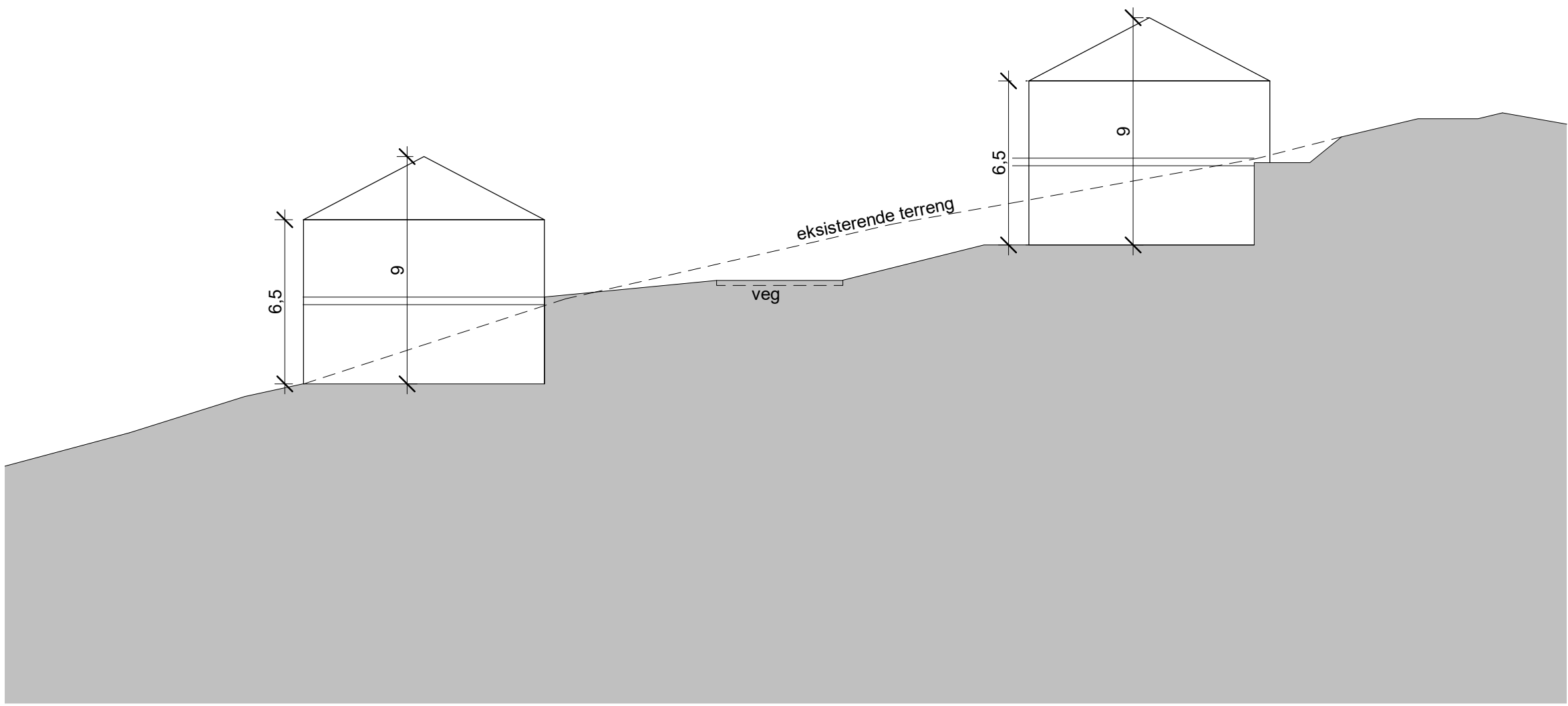
Prinsippsnitt terrengtilpassning 1 : 200
